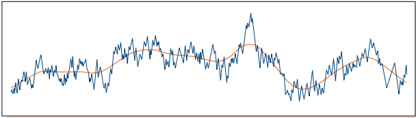
> Bild 1: Den primära profilen och medellinjen för den primära profilens ( \lambda_c cut-off) filter
