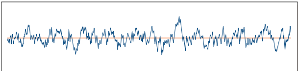
> Bild 2: Ytjämnhetsprofilen med dess medellinje (högpasfiltering av den primära profilen med en cut-off-våglängd på \lambda_c )
