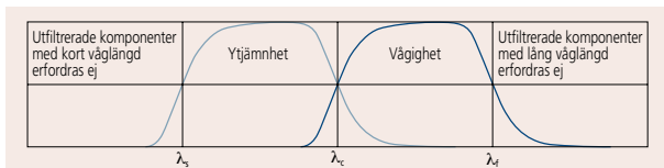
> Bild 5: Överföringsparametrar för de filter som används för att separera egenskaperna för ytjämnhet och vågighet. Filterrespons är Gaussian enligt EN ISO 11562: 1998
